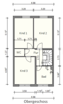
Grundriss OG
