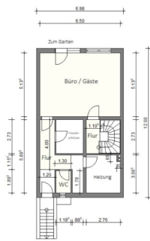
Grundriss KG
