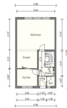
Grundriss EG
